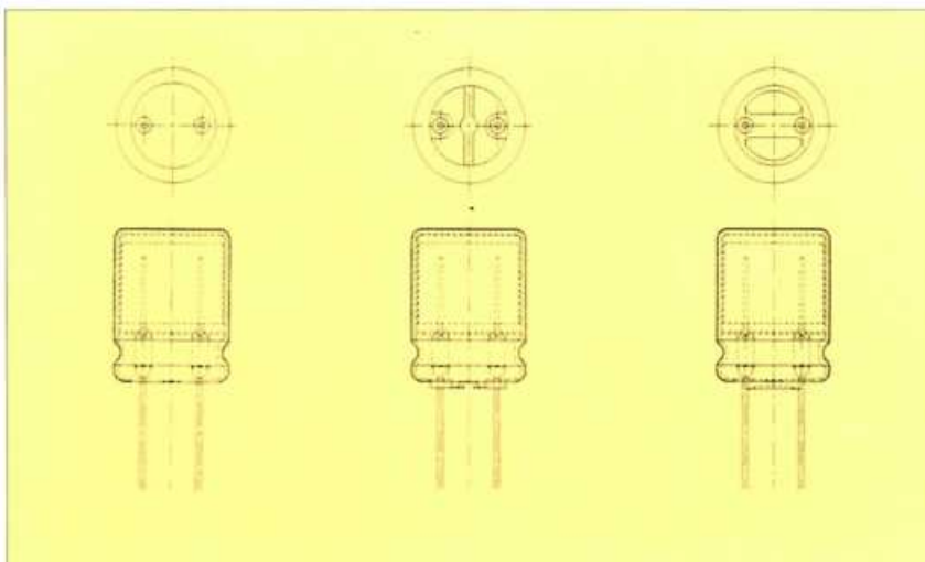
De gladde rubberen afsluitschijf (links) wordt vervangen door een geprofileerd type (rechts).
