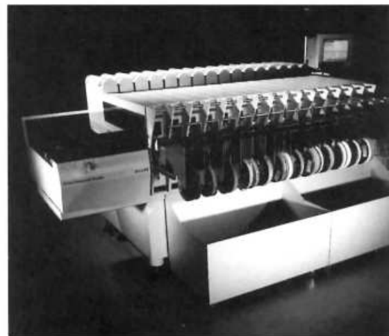
De nieuwe Fast Component Mounter (FCM).
