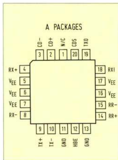
Afb. 2 De nieuwe PLCC-omhulling van de NE83Q92A20.
